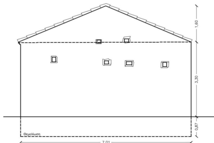
ΑΝΑΤΟΛΙΚΗ ΟΨΗ
