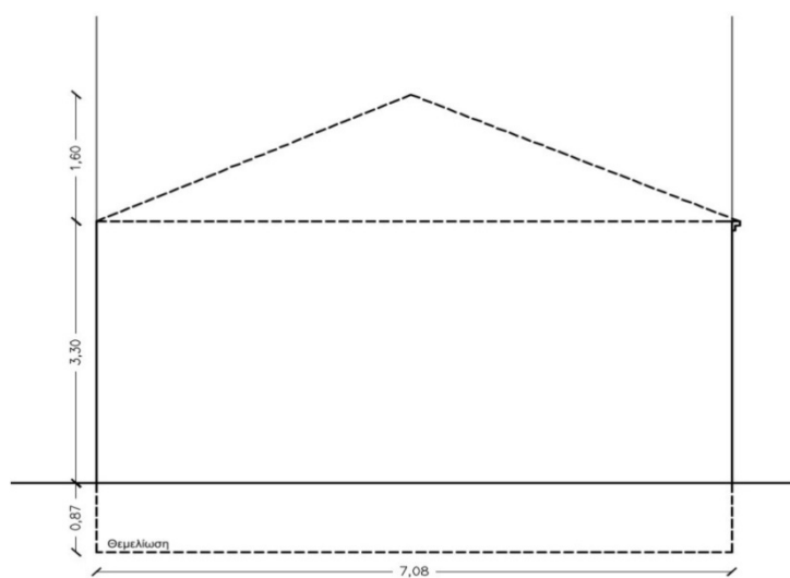
ΔΥΤΙΚΗ ΟΨΗ (ΜΕΣΟΤΟΙΧΙΑ)
