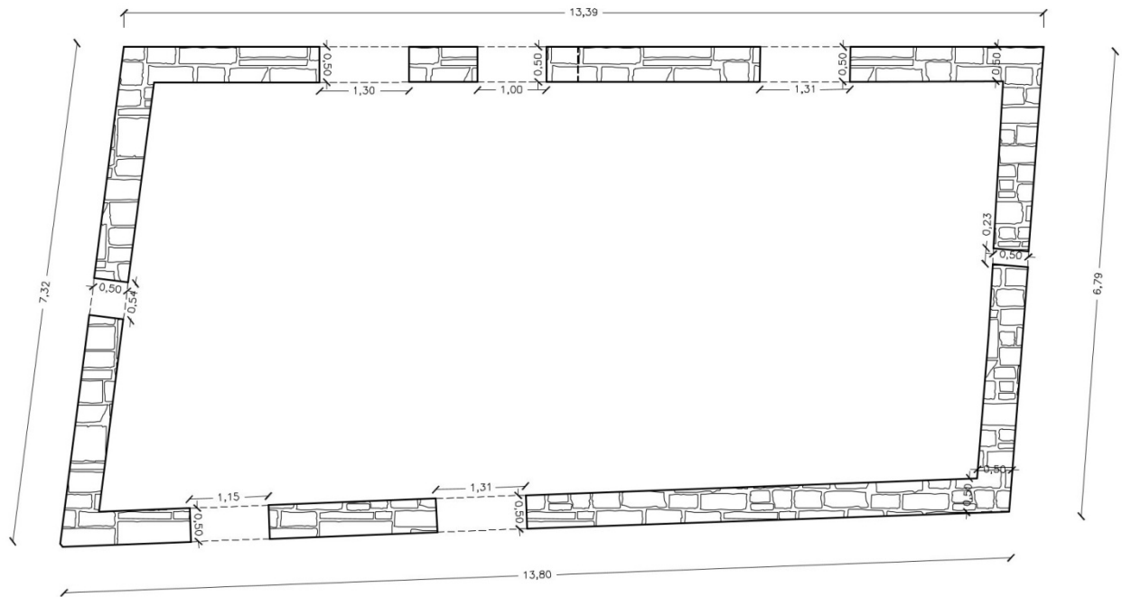
ΚΑΤΟΨΗ ΙΣΟΓΕΙΟΥ
