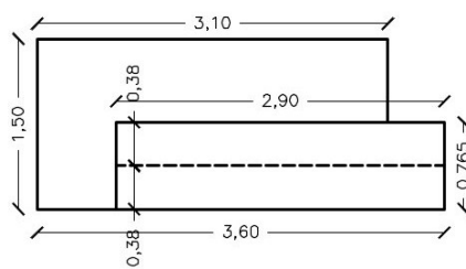
ΚΑΤΟΨΗ
